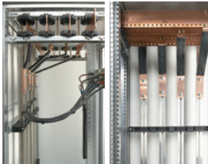
Подключение к главным горизонтальным шинам должно выполняться индивидуально. Для этого идеально подходят гибкие шины.
