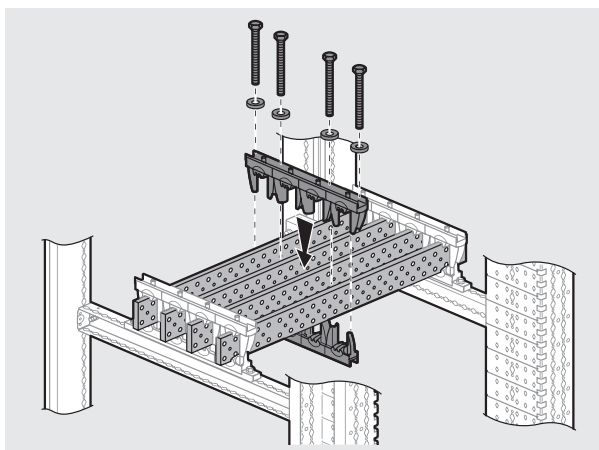
Дополнительный суппорт Кат. № 0 373 23 в сборе
