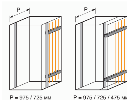
Сбоку в шкафу + позади монтажных стоек
