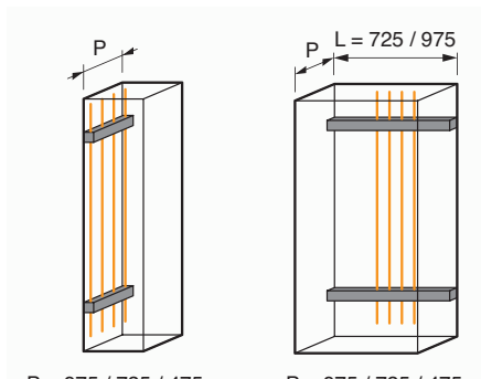
Сбоку в наружной кабельной секции
