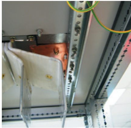
Элемент подачи питания: крепление с траверсами с усилителем верхней панели.
