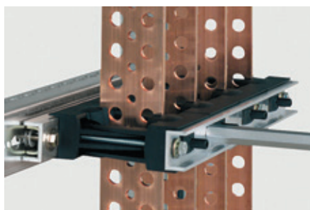
Вставьте шины в съёмную часть изолирующих суппортов (момент затяжки 7 Н·м): плоские шины Кат. №№ 0 374 40/41/43/46/59
