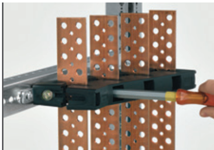
Вставьте шины в съёмную часть изолирующих суппортов (момент затяжки 7 Н·м) – плоские шины Кат. №№ 0 374 40/41/43/59 ...
