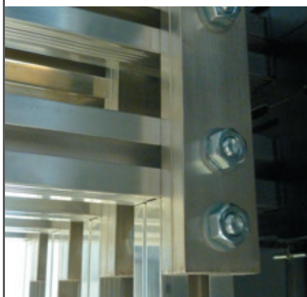
Соединение между алюминиевыми вертикальными и горизонтальными двойными главными шинами, созданное с помощью алюминиевых шин.
