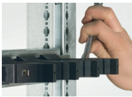
Прикрепите суппорт винтами М6. (момент затяжки 10 Н·м)
