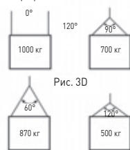
Рис. 3В - Подъём щита стропами за угловые профили
