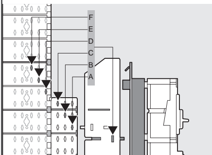
Комбинируя монтажные стойки и накладки Кат. № 0 207 50, можно получить 6 позиций по глубине.
