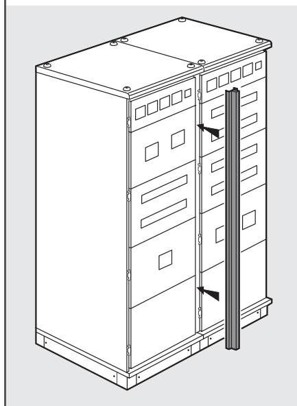
Между дверями устанавливается декоративный профиль Кат. № 0 205 65 для шкафов высотой 2000 мм и Кат. № 0 208 47 для шкафов высотой 2200 мм.
