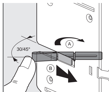
Установка пружин
