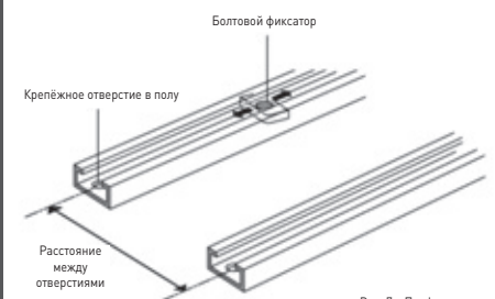
Рис. 7 - Профили С-образного сечения
