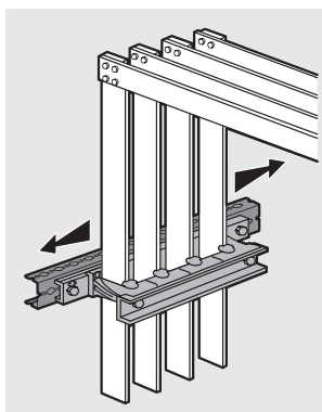
Траверсы Кат. №№ 0 205 51/52/53 позволяют смещать положение шин на 5 мм, что облегчает подсоединение вертикальных шин к горизонтальным.
