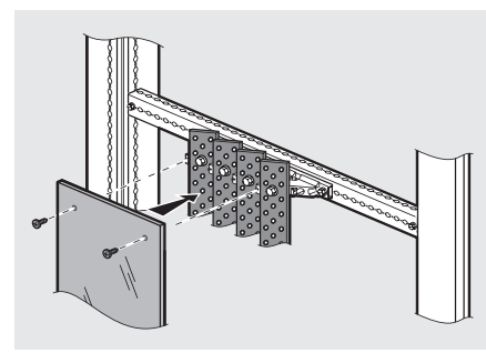
На суппорт можно надеть защитную крышку (в комплект не входит) и закрепить 2 прилагаемыми винтами
