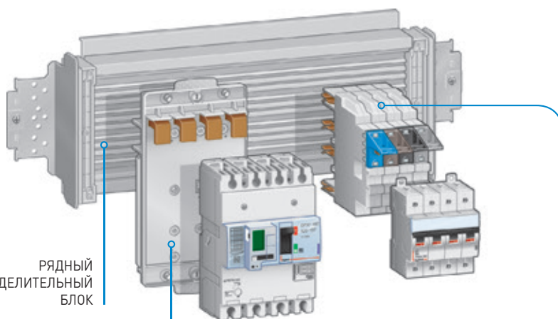
КОНТАКТНЫЕ ОСНОВАНИЯ АВТОМАТИЧЕСКИХ ВЫКЛЮЧАТЕЛЕЙ DPX 3 Для крепления и подключения 3П и 4П автоматических выключателей DPX 3 160 и 250, и АВДТ.
