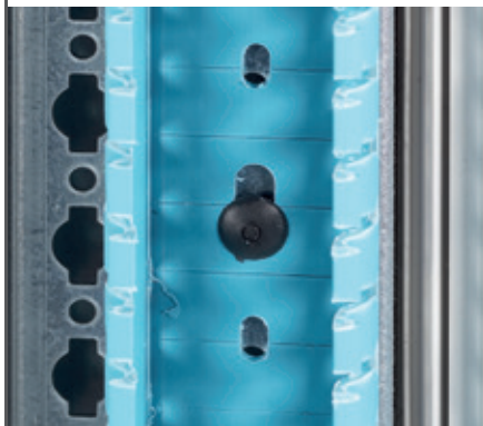
Для крепления лотков Lina 25 используются заклёпки Кат. № 0 200 80.
